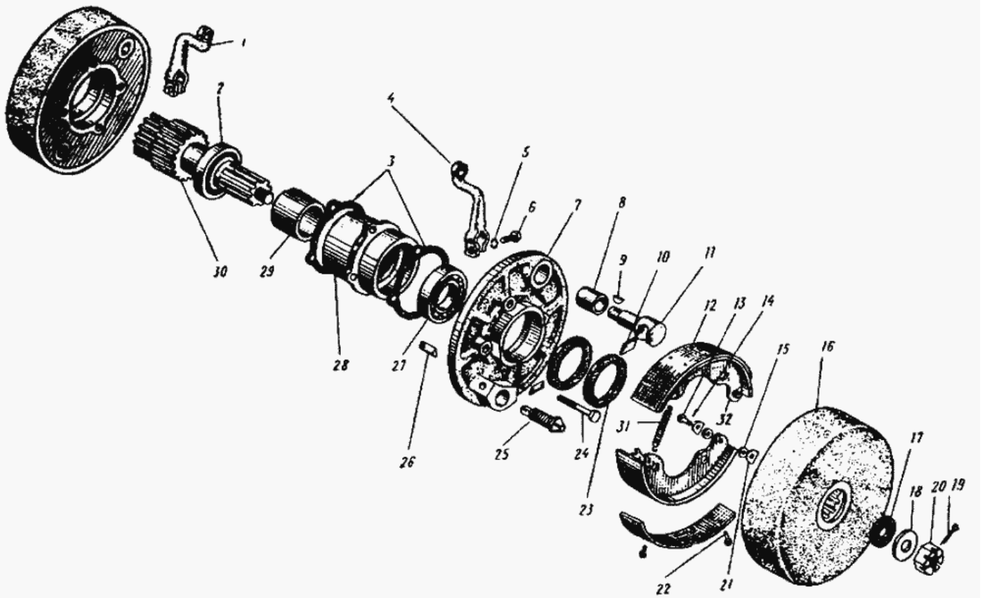
Рис. 42. Тормоза и тормозные барабаны
